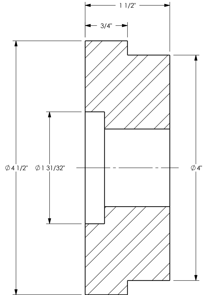
SECTION A-A
